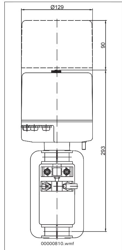
Fig. 176 actuator baelz 373-E02-S21
