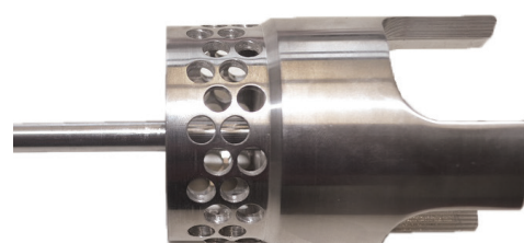
bælz 340-2-B cage plug
